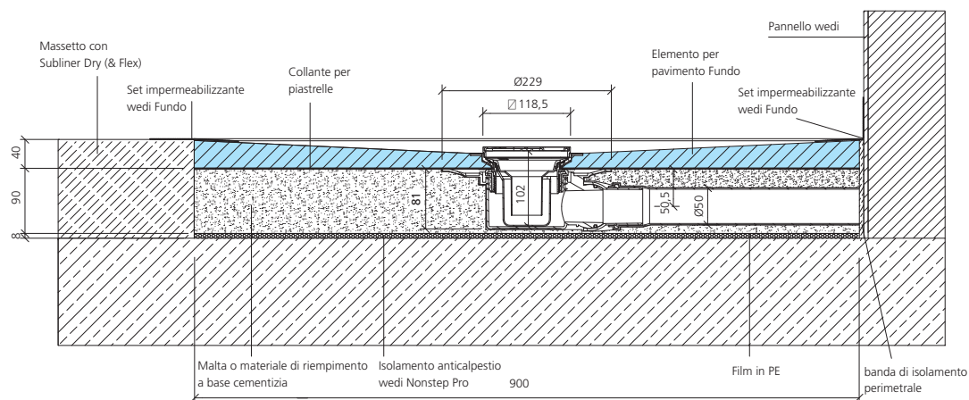
Scarico Fundo orizzontale, DN 50, pavimento con massetto
