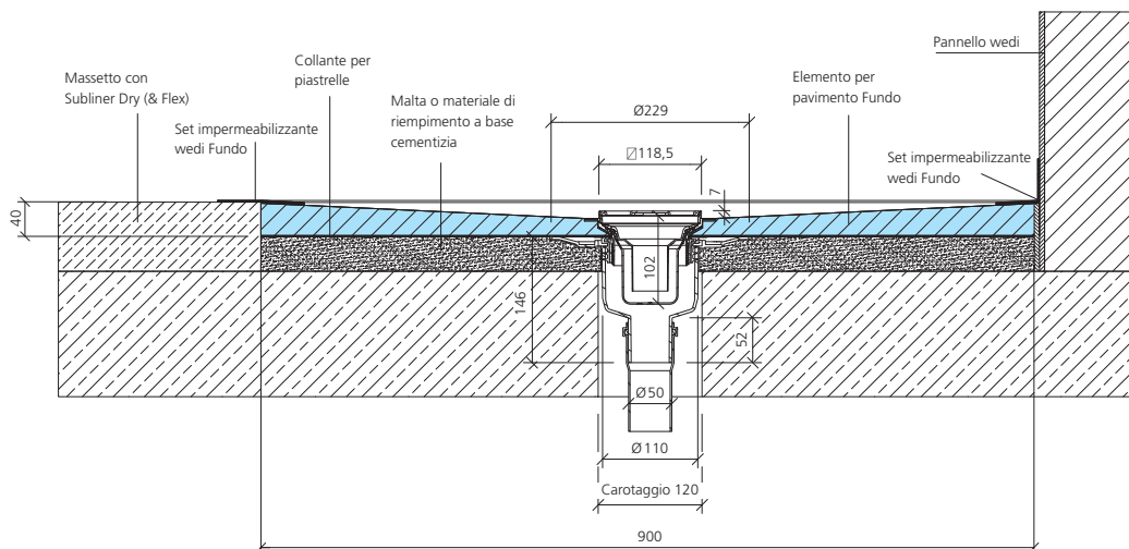
Scarico Fundo verticale, DN 50, pavimento con massetto
