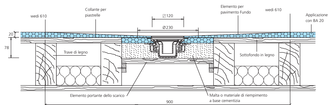
Scarico Fundo Mini Max, DN 40, su pavimento in legno
