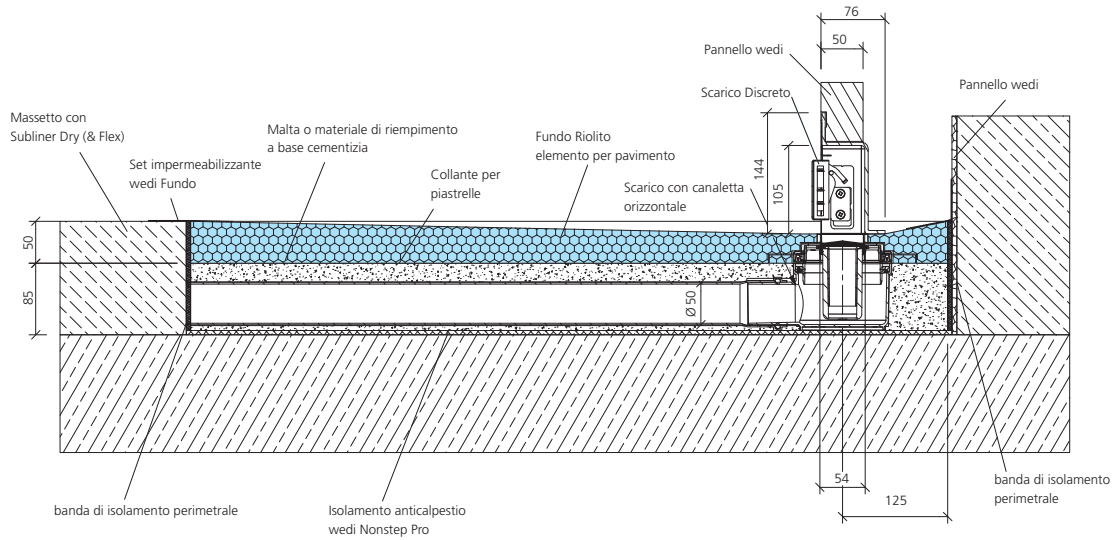
Fundo Discreto, scarico a parete, DN 50, pavimento con massetto
