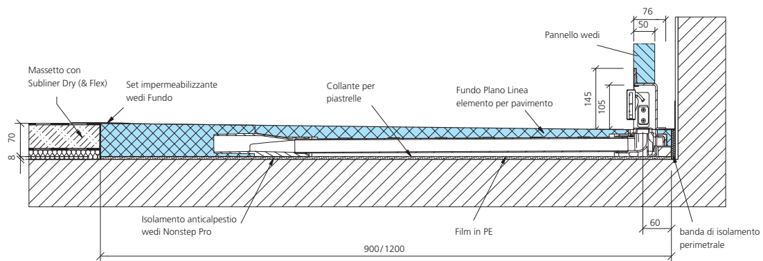
Fundo Discreto, scarico a parete, DN 40, pavimento con massetto
