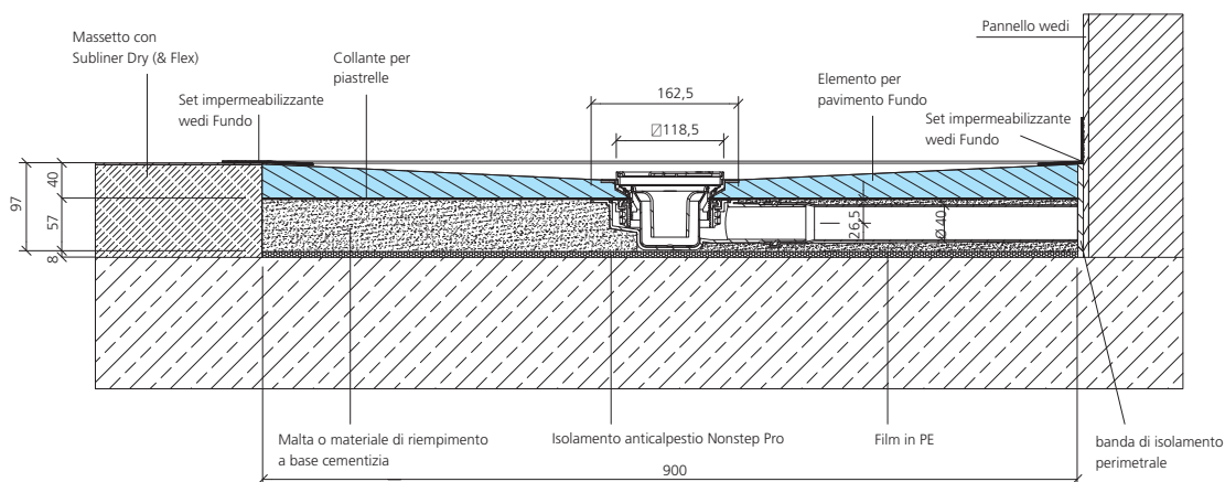
Scarico Fundo Mini Max, DN 40, pavimento con massetto
