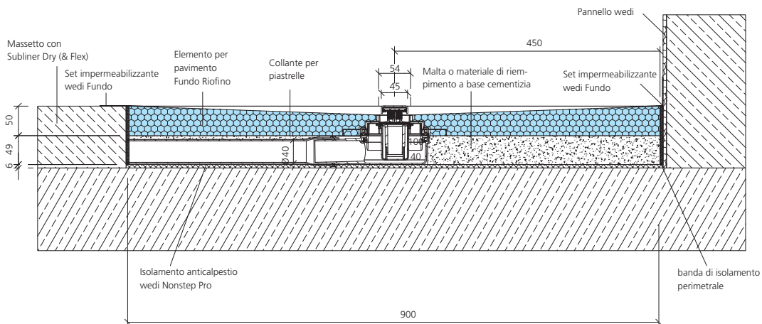
Scarico Fondo Riofino Mini Max, DN 40, pavimento con massetto
