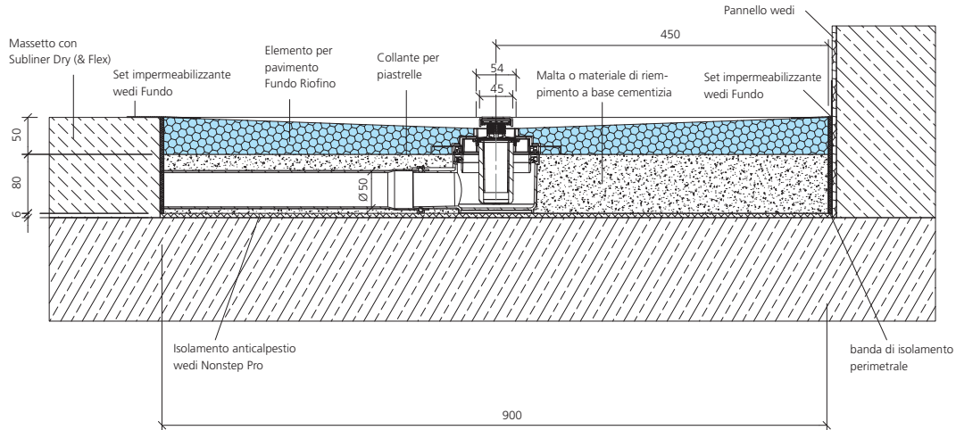
Scarico Fundo Riofino orizzontale, DN 50, pavimento con massetto
