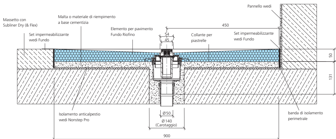
Scarico Fondo Riofino verticale, DN 50, pavimento con massetto
