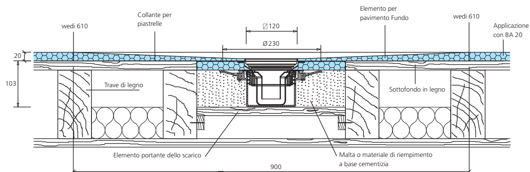
Scarico Fundo orizzontale, DN 50, su pavimento in legno
