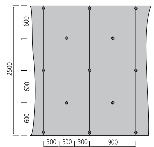
Anwendung vollflächige Verklebung und Verdübelung für BA 12,5; BA 20; BA 30; BA 50 mm.
