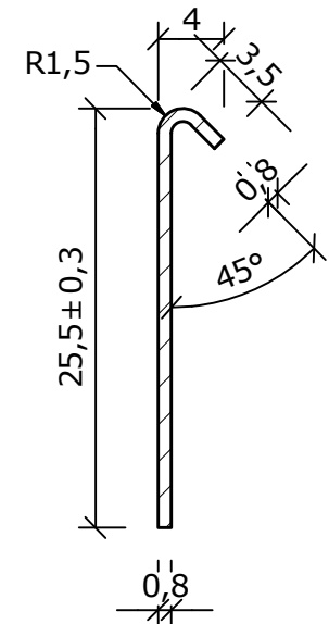
section A-A (2 : 1)
