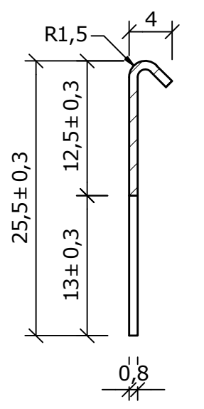
section B-B (2 : 1)
