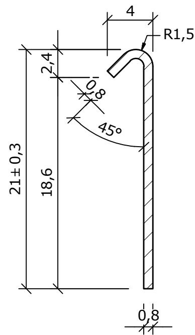
section A-A (3 : 1)
