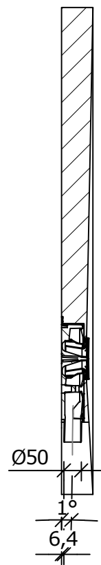
Schnitt B-B (1 : 15)
