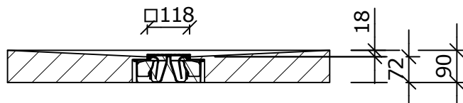
Schnitt A-A (1 : 15)
