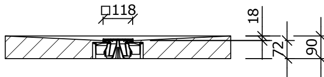
Schnitt A-A (1 : 15)
