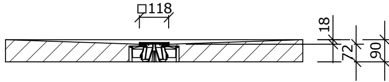
Schnitt A-A (1 : 15)
