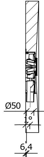
Schnitt B-B (1 : 15)
