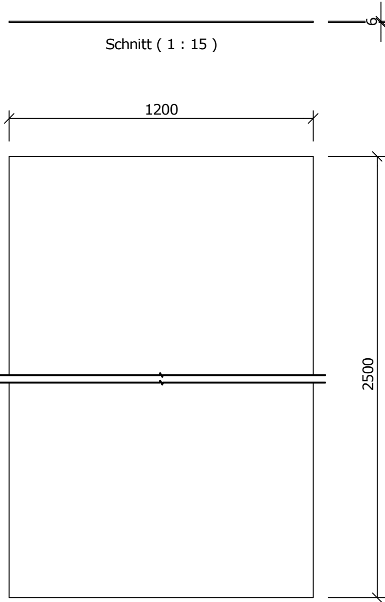
Draufsicht ( 1 : 15 )
