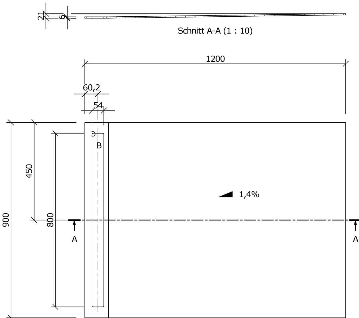
Draufsicht ( 1 : 10 )
