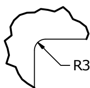
Detail B ( 1 : 1 )
