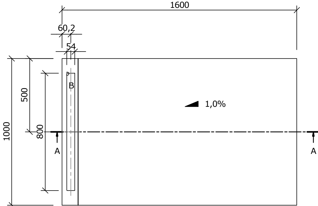
Draufsicht ( 1 : 15 )
