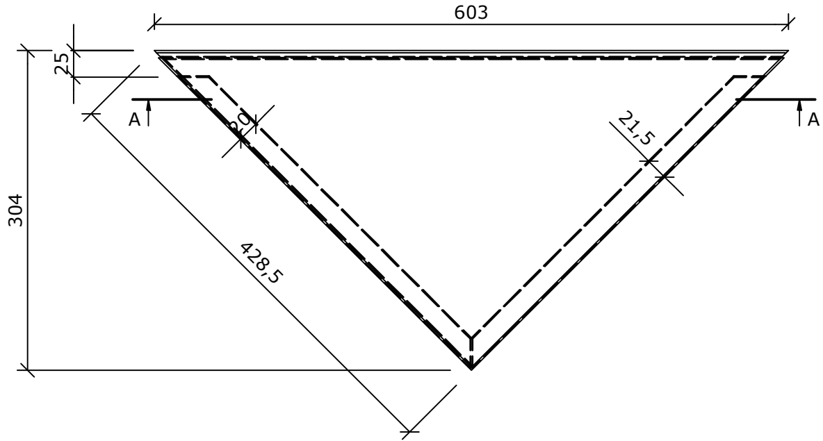
Draufsicht (1 : 5)
