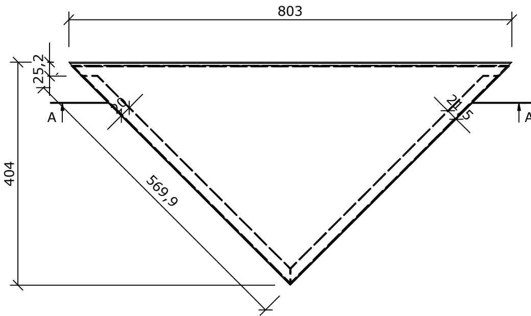
Draufsicht (1 : 7)
