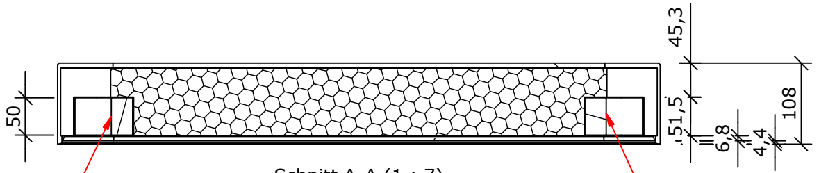
Schnitt A-A (1 : 7)
